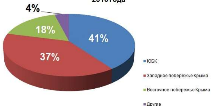
Распределение туристов по регионам Крыма с начала 2016 года
